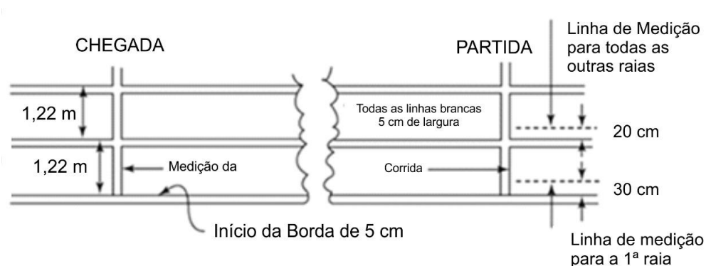
Figura da RT 14 Medidas da Pista (Vista do campo interno)
