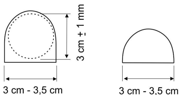
Figura da RT 26 Ponteiras alternativas para Barra Transversal
